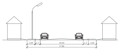
поперечный профиль улиц шириной 17 м
