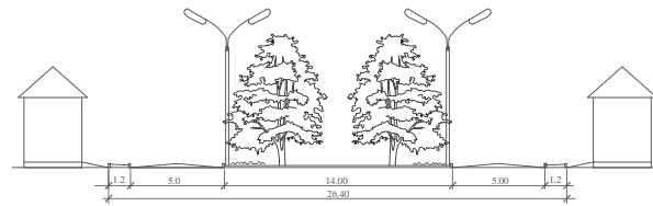
поперечный профиль улиц шириной 26,4 м
